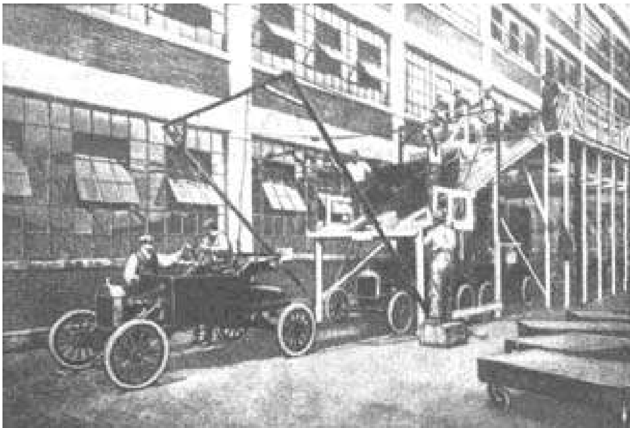
Сборка автомобилей на заводе Форда. Фотография. 1913 г.
