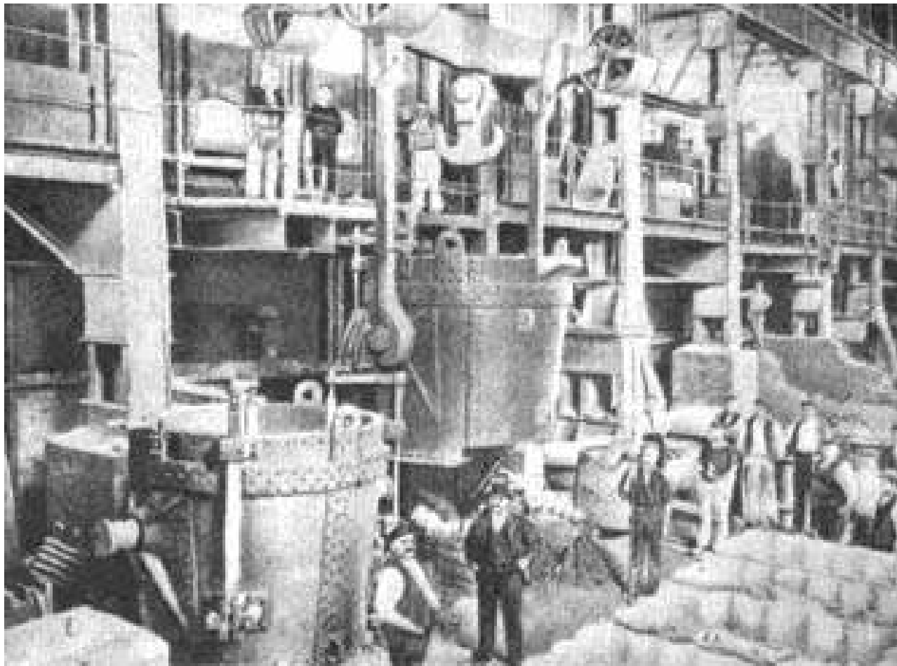
Мартеновский цех завода фирмы Виккерс (Англия). Фотография. 1884 г.
